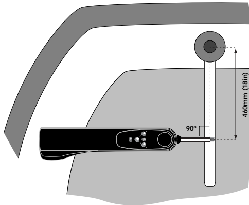
Abb. 5.2 - Installation, Aufsicht
