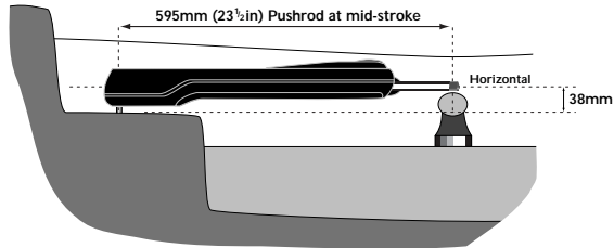
Abb. 5.1 - Installation, Seitenansicht
