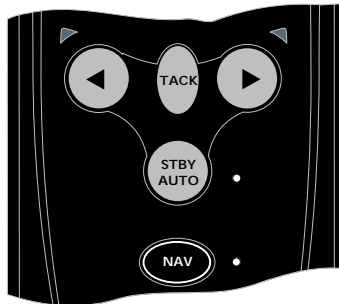
Abb. 3.1 - Nav-Modus aktivieren
