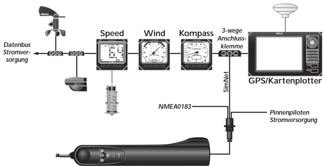
Abb. 5.7 - Typische SimNet Installation
