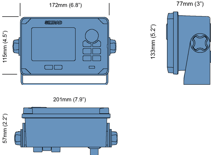
8.1 - AI50 dimensions
